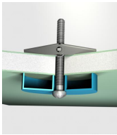
Cheville à ressort - vue en coupe
